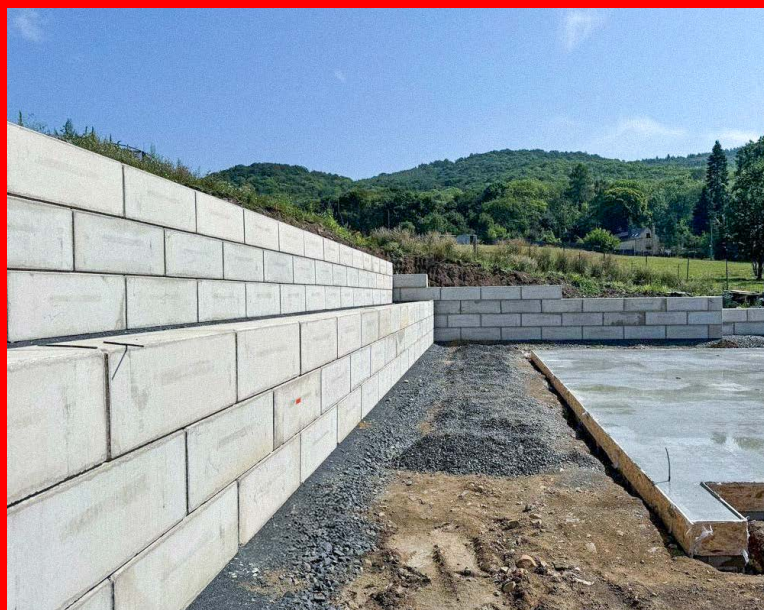
Opěrná zeď svahu u RD
